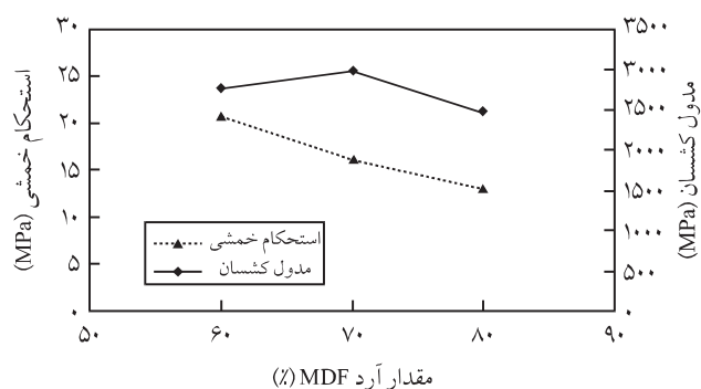
شکل ۱- اثر مقدار آرد MDF بر مدول کشسان و استحکام خمشی کامپوزیت‌های چوب - پلاستیک.
