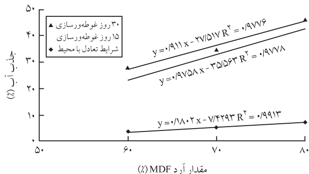
شکل ۲- رابطه بین درصد جذب آب و مقدار آرد MDF در کامپوزیت‌های چوب - پلاستیک.
