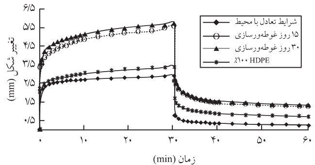
شکل ۴- اثر زمان غوطه‌ورسازی بر خزش کامپوزیت‌های چوب - پلاستیک (مقدار ۶۰٪ آرد MDF).
